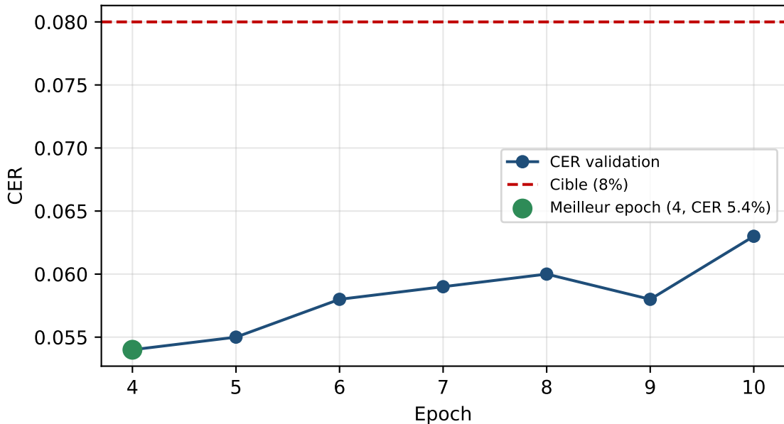
Taux d'erreur caractère (validation) par epoch
