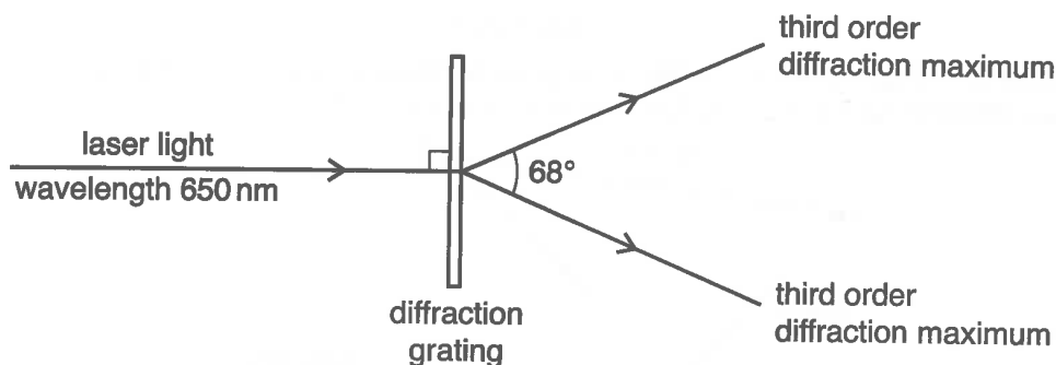
Fig. 4.1 (not to scale)
