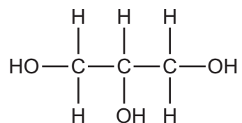
propane-1,2,3-triol
