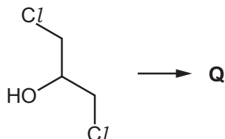
1,3-dichloropropan-2-ol
