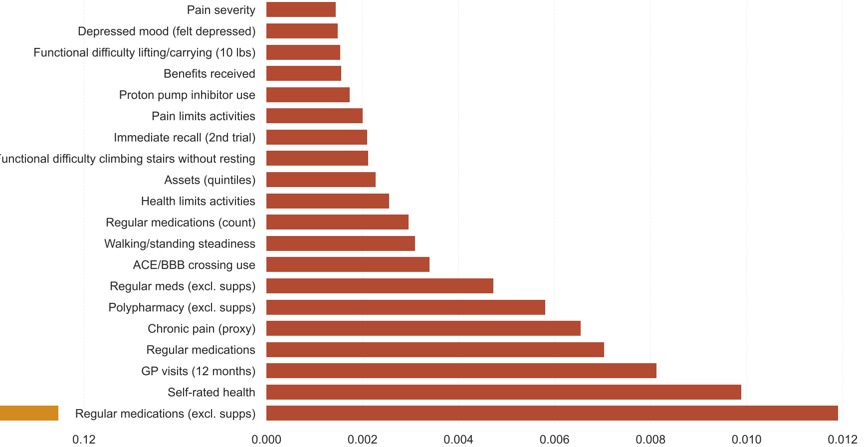
MLP
