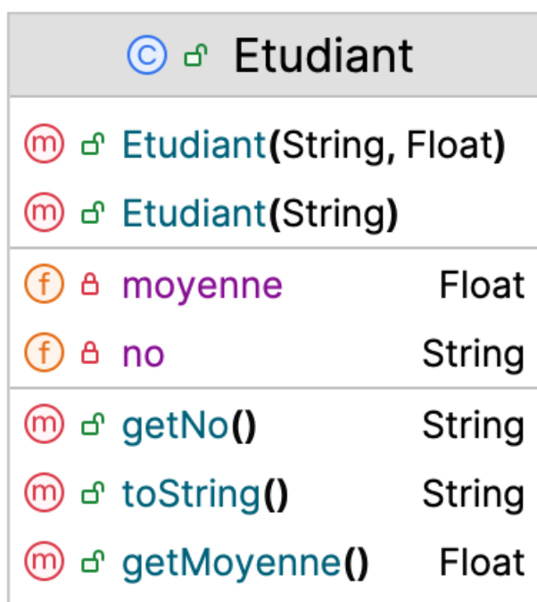
Figure 2.1. Classe Etudiant
