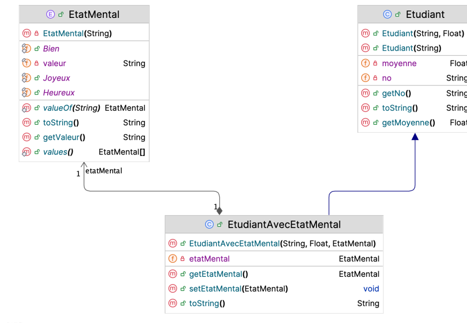
Figure 2.3. EtudiantAvecEtatMental
