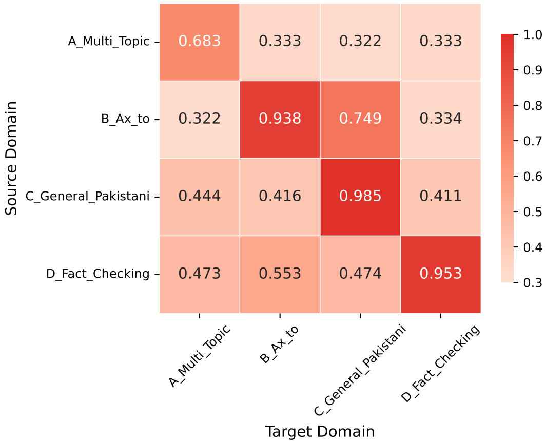
Cross-Domain F1 Performance Matrix: Nastaliq Fake News (XLM-R Base)
