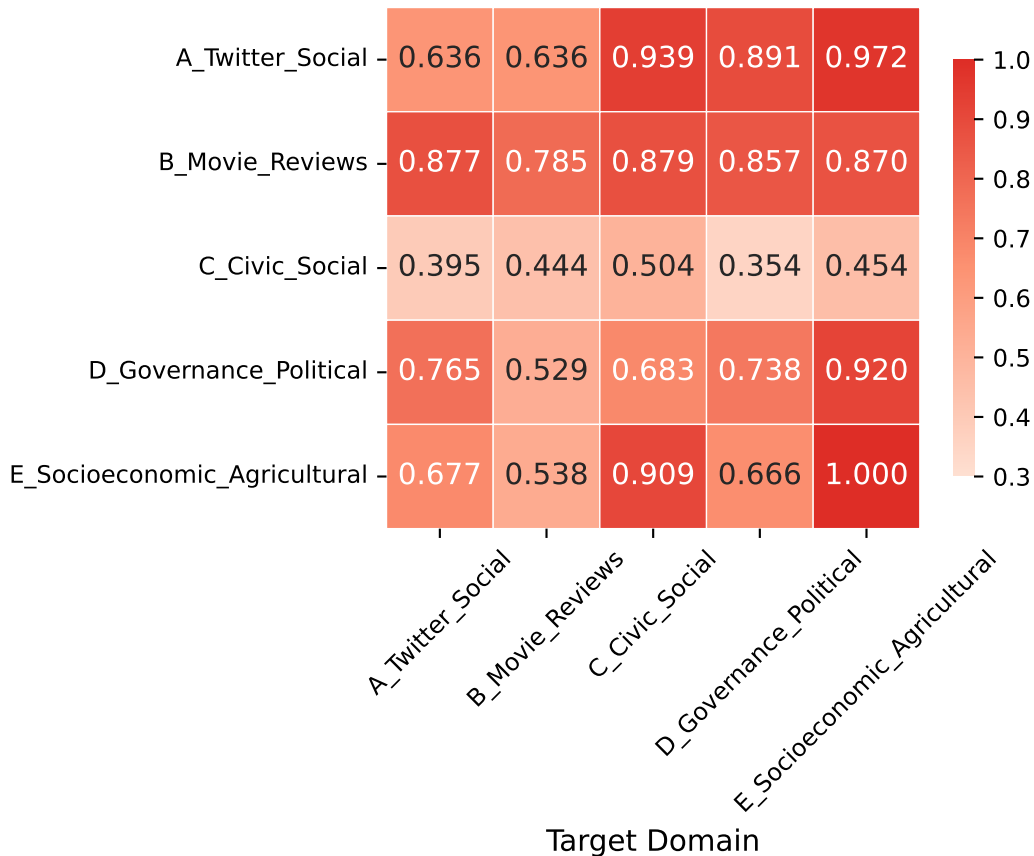
Cross-Domain F1 Performance Matrix: Nastaliq Sentiment (XLM-R Base)
