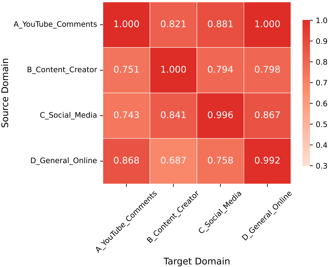
Cross-Domain F1 Performance Matrix: Roman Cyber Abuse (XLM-R Base)
