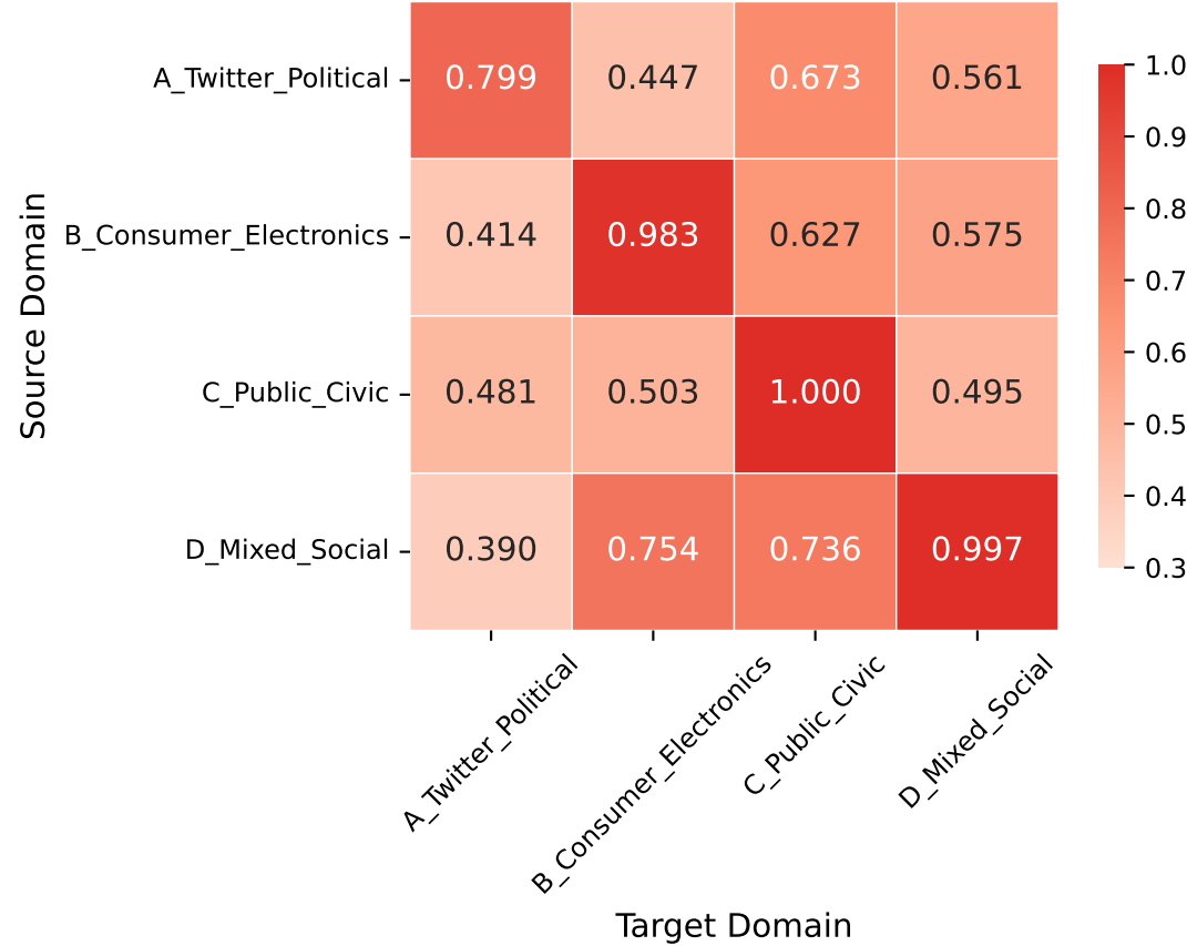
Cross-Domain F1 Performance Matrix: Roman Twitter Opinions (XLM-R Base)
