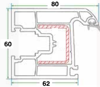
بروفائل ضلفة شبك وياپ سحاب 60 Sliding Sash Profile 60
