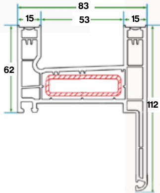
بروفائل الفريم سحاب مع حاجب 60 Sliding Fringed Frame Profile 60
