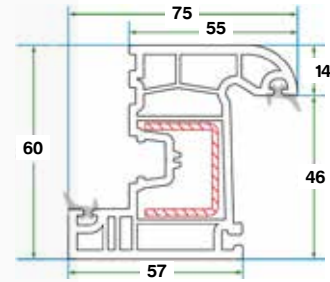
بروفايل ضلفة الشباك 60 Sash Profile 60
