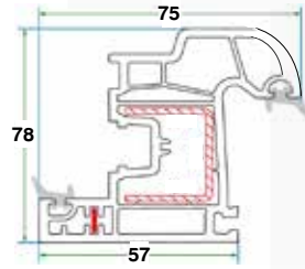
بروفايل ضلفة الشباك 80 Sash Profile 80
