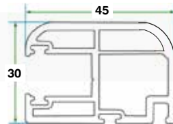
بروفائل ضلفة مانع الذباب سحاب 60 Sliding Fly Screen Sash Profile 60
