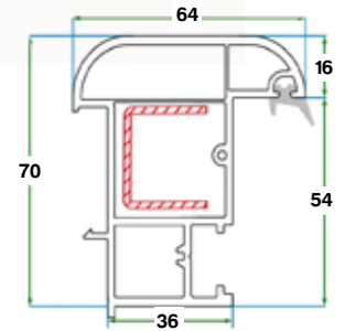
بروفايل القائم الوسطي المتحرك 70 Movabel Mullion Profile 70
