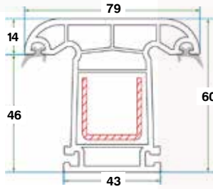
بروفايل القائم الوسطي 60 + سحب MULLION PROFILE 60 +SLIDING
