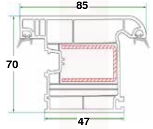
بروفايل ضلفة الشباك للخارج 70 window Sash Profile 70 (opening out)
