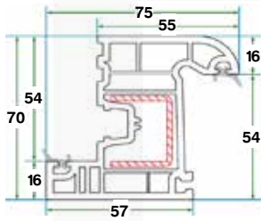
بروفايل ضلفة الشباك 70 Sash Profile 70
