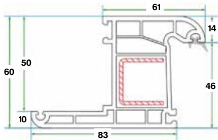
بروفايل الفريم مع حاجب 60 Fringed Frame Profile 60
