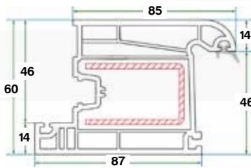
بروفايل ضلفة الباب للداخل 60 Door Sash Profile 60 (opening in)
