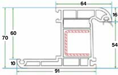
بروفايل الفريم مع حاجب 70 Fringed Frame Profile 70
