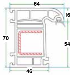
بروفايل الفريم بدون حاجب 70 Frame Profile 70
