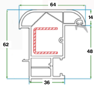
بروفايل القائم الوسطي المتحرك 60 Movable mullion profile 60
