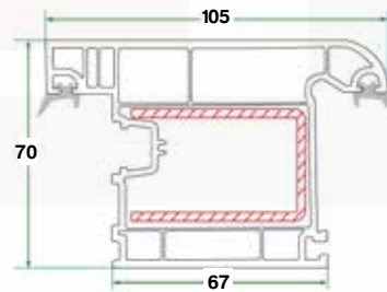
بروفايل ضلفة الباب للخارج 70 Door Sash Profile 70 (opening out)
