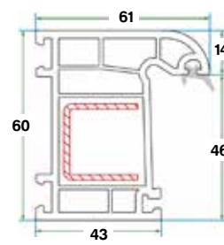
بروفايل الفريم بدون حاجب 60 Frame Profile 60
