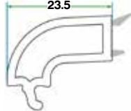
بروفائلات لاقط زجاج دبل Double Glazing Bead 20/24 mm
