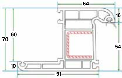
بروفايل الفريم مع حاجب Fringed Frame Profile 70
