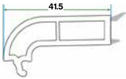
بروفائلات لاقط زجاج مفرد Single Glazing Bead
