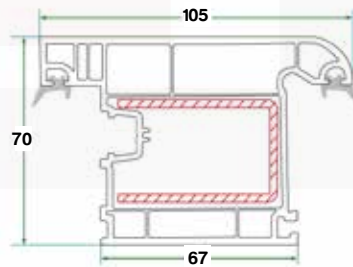
بروفايل ضلفة الباب للخارج Door Sash Profile 70 (opening out)
