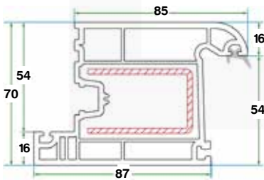
بروفايل ضلفة الباب للداخل Door Sash Profile 70 (opening in)
