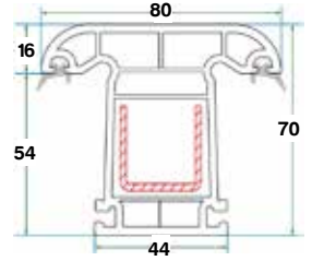
بروفايل القائم الوسطي MULLION PROFILE 70
