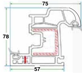
بروفايل ضلفة الشباك Sash Profile 80
