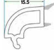
بروفائلات لاقط زجاج ثلاثي Tripple Glazing Bead
