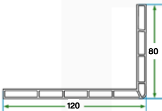
بروفائلات برواز زاوية Casing profile
