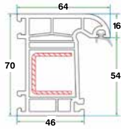
بروفايل الفريم بدون حاجب Frame Profile 70
