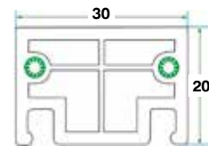
بروفايل القائم الوسطي لمانع الذباب سحاب 60 Fly Screen Sliding Mullion Profile 60
