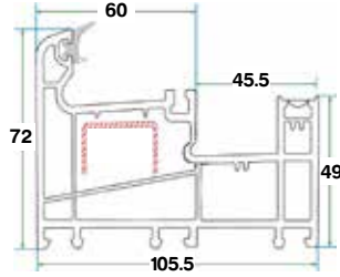
بروفايل الفريم ثابت سحاب 60 Sliding Fix Frame Profile 60
