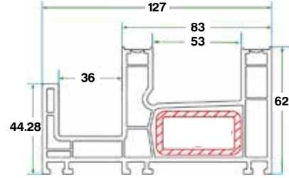
بروفايل سحاب مع مانع ذباب 60 Flyscreen sliding Frame Profile 60
