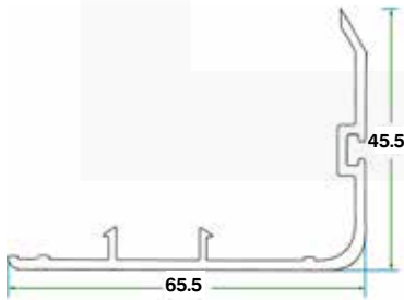
بروفايل اغلاق القفل سحاب 60 Sliding Interlock Profile 60
