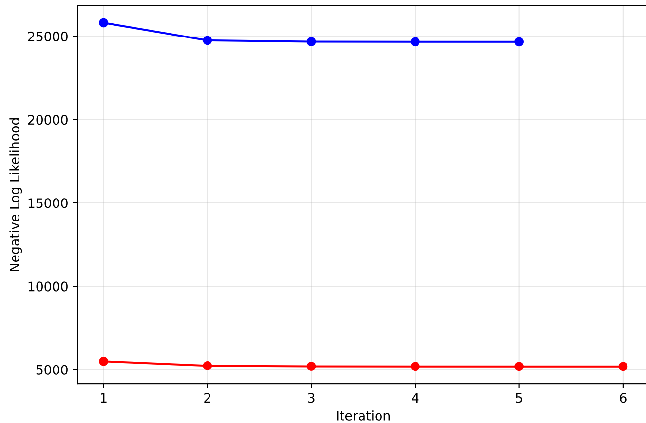
NLL
