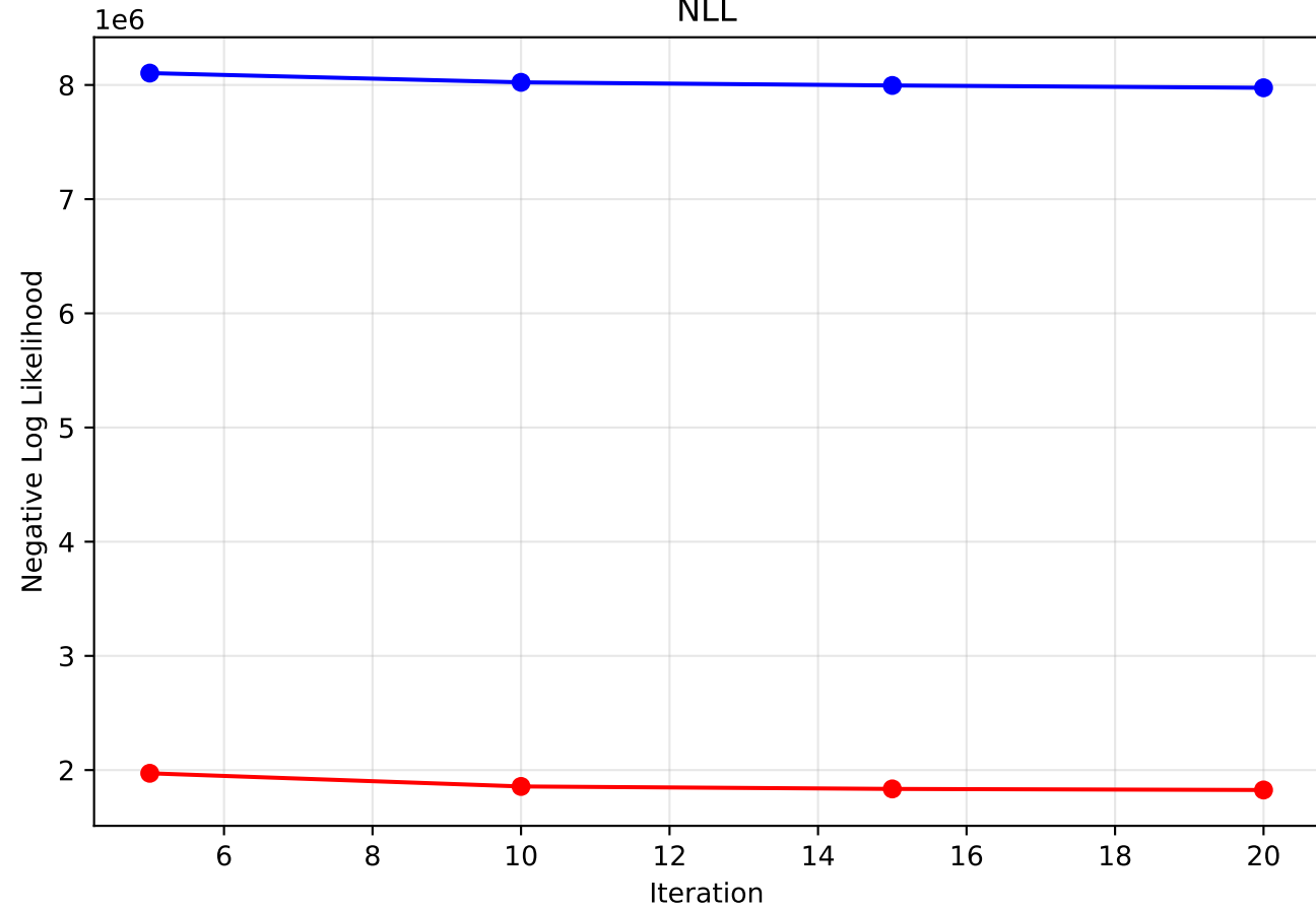
NLL
