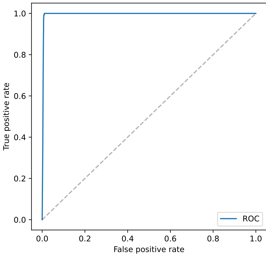
ROC (test, n=1845)
