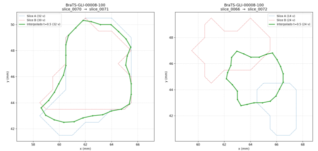
Figura 1. Caso BraTS-GLI-00008-100 con las mejoras de pre-alineación activas. Izquierda: slices consecutivos 0070 → 0071, k^* = 0 . Derecha: slices separados por 6 cortes, 0066 → 0072, k^* = 1 . Ambos resueltos sin auto-intersecciones.
