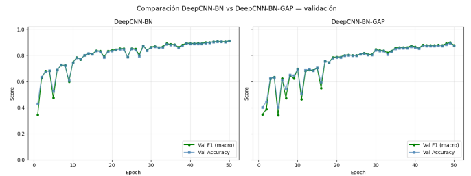
Figura 18: Comparación del F1-Macro de validación entre DeepCNN-BN y DeepCNN-BN-GAP a lo largo del entrenamiento.
