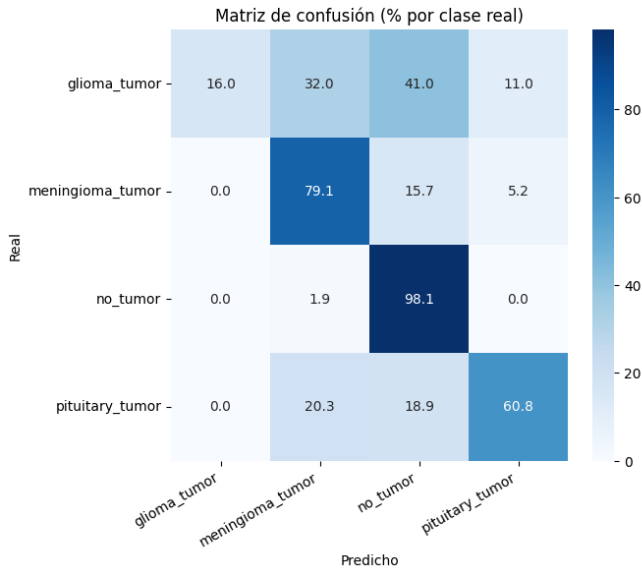
Figura 11: Matriz de confusión normalizada de DeepCNN-BN (cabecal FC) sobre Testing .
