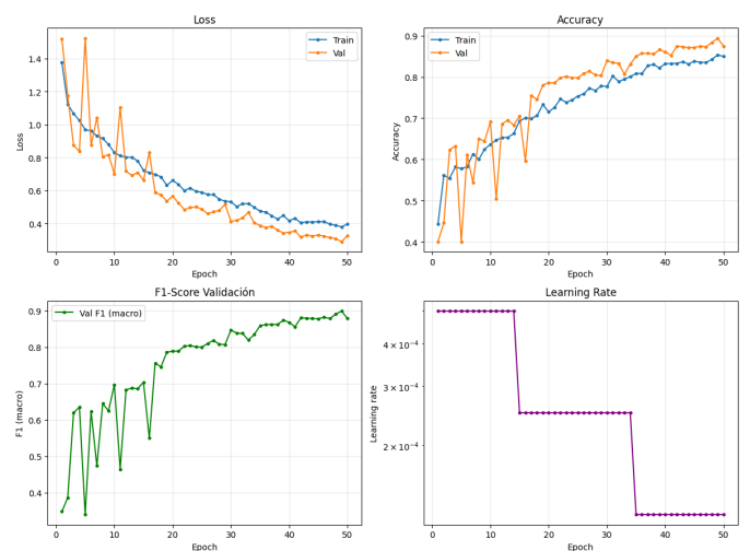
Figura 17: Curvas de entrenamiento de DeepCNN-BN-GAP.
