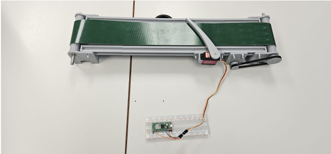
Figure 5: Construcción de la cinta transportadora.
