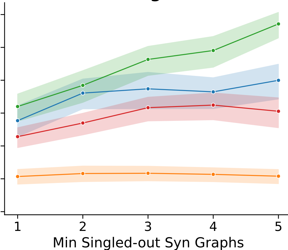
Dataset: Ego-Twitter
