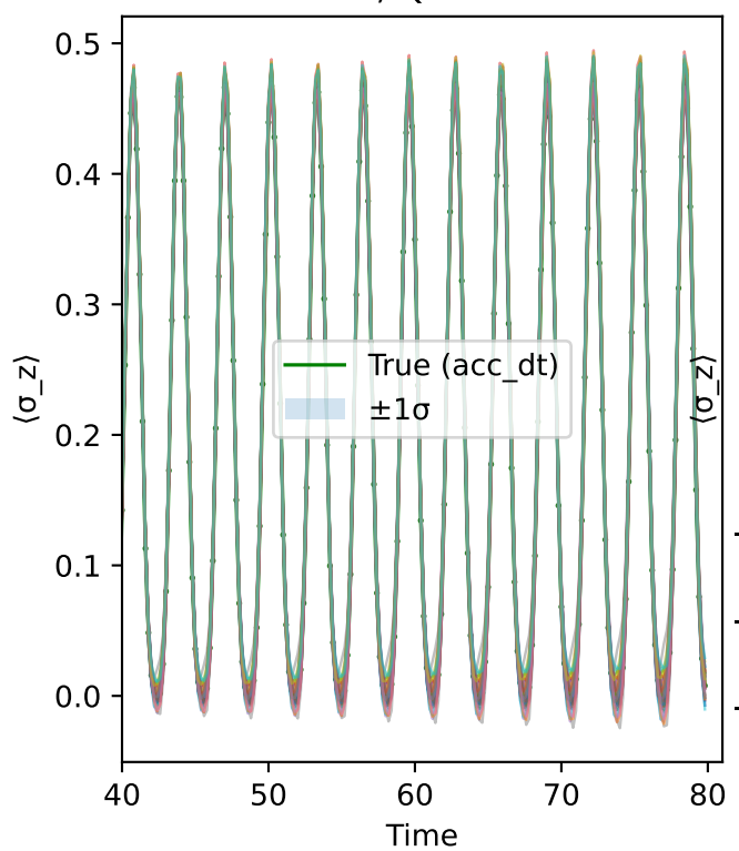
N=4, Qubit=1
