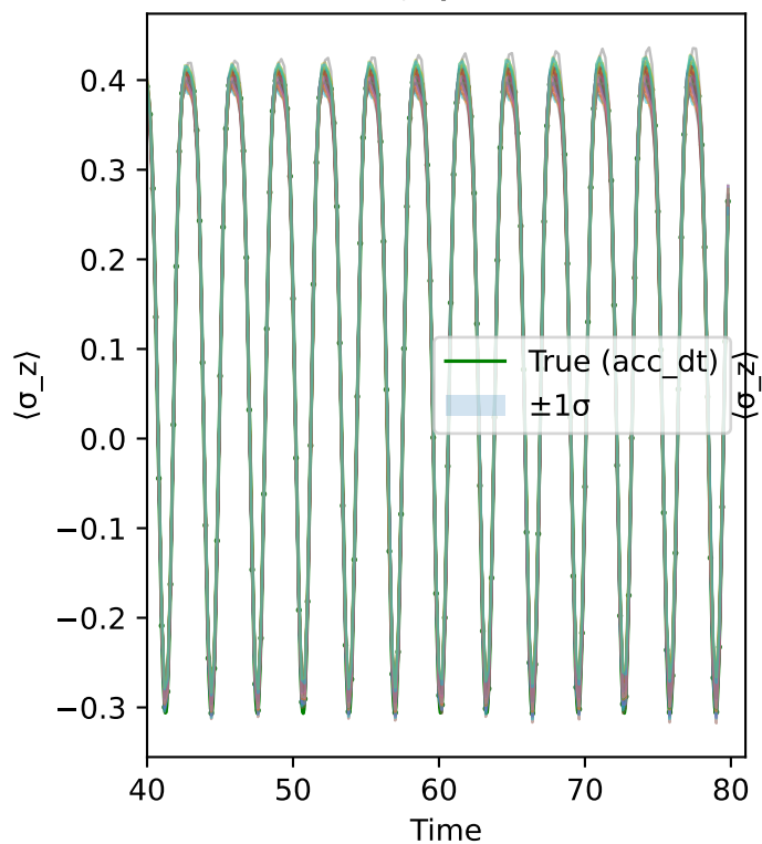
N=4, Qubit=1
