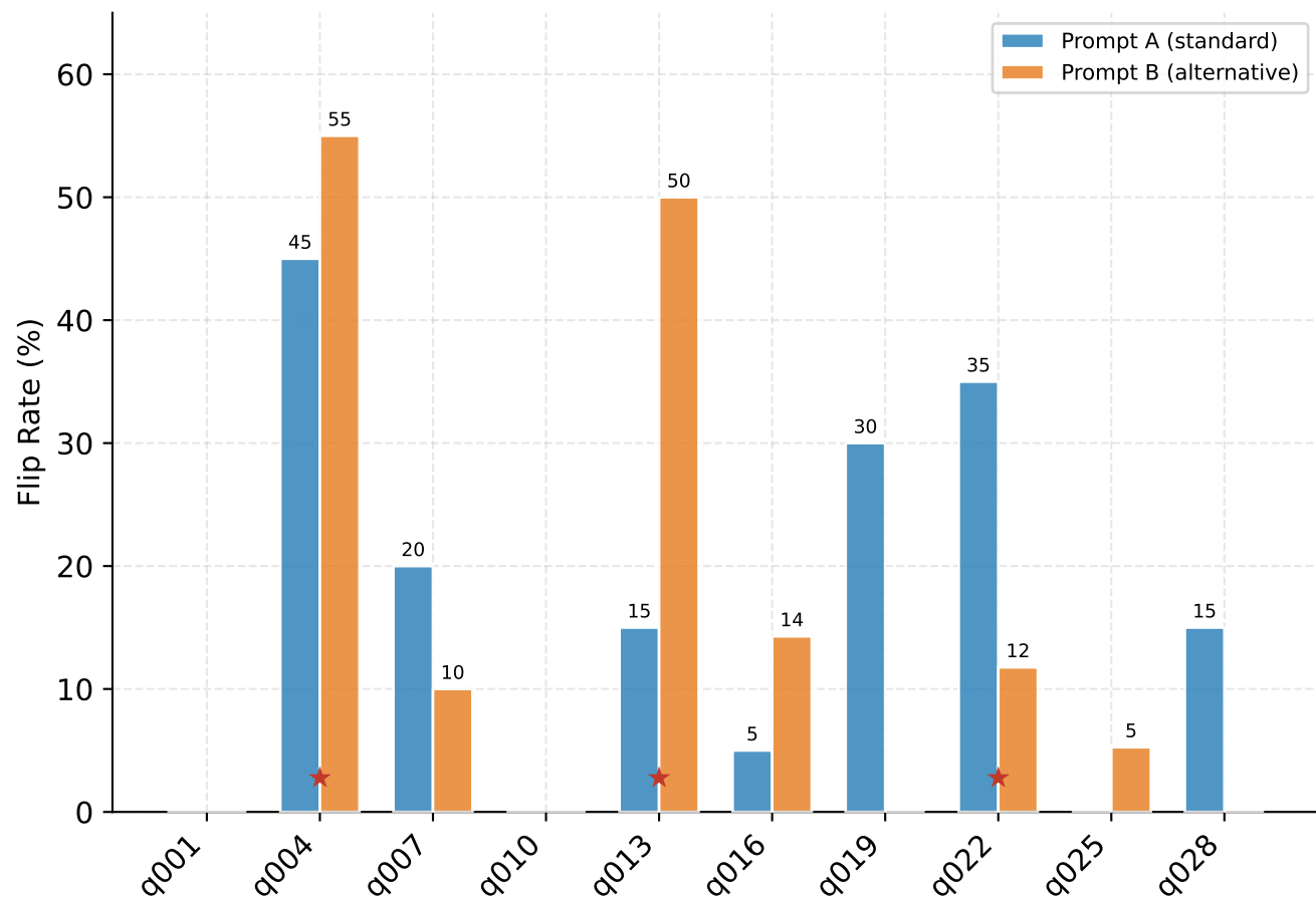
GPT-4.1-mini
