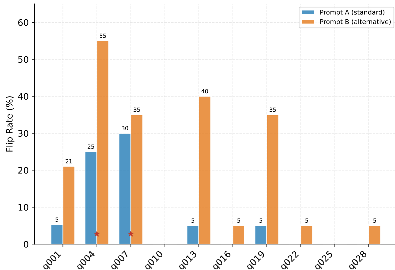
GPT-4o-mini
