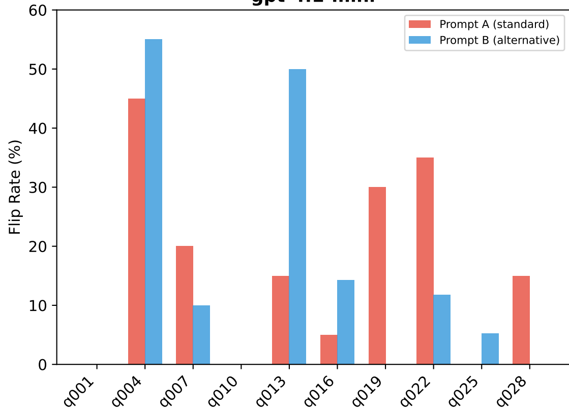
gpt-4.1-mini
