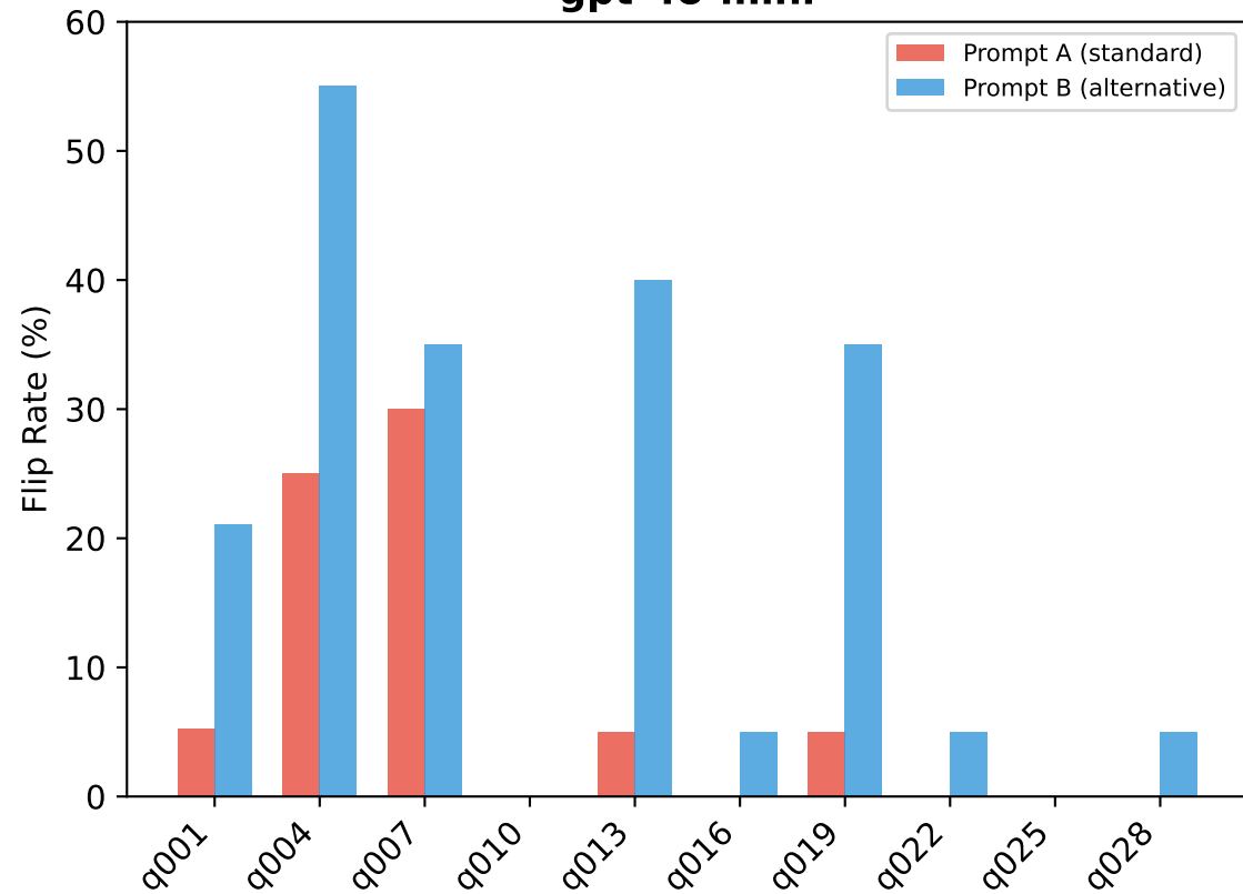
gpt-4o-mini
