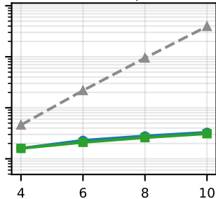
Heat Eqn
