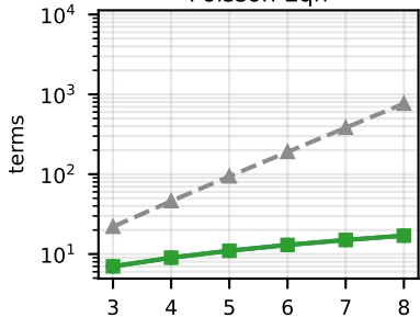
Poisson Eqn
