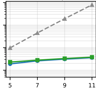
Wave Eqn
