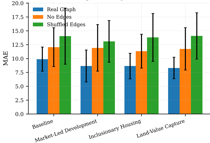
Degradation per scenario
