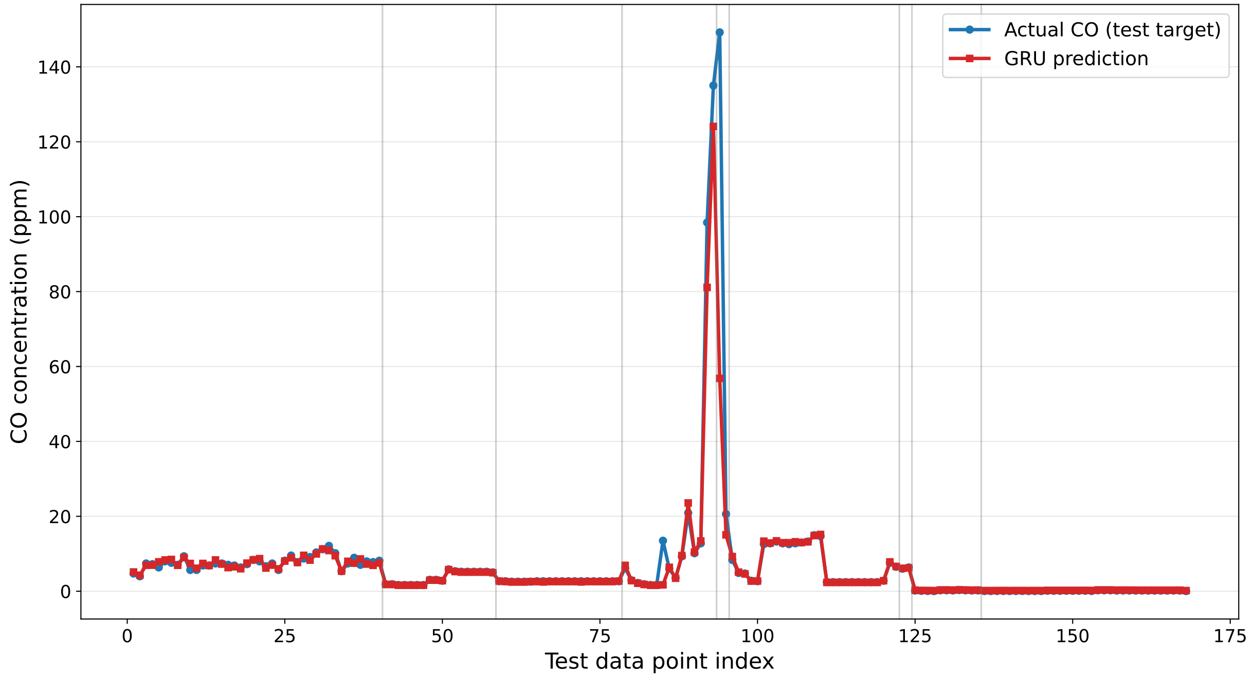
GRU CO Forecast: Actual vs Predicted Test Data
