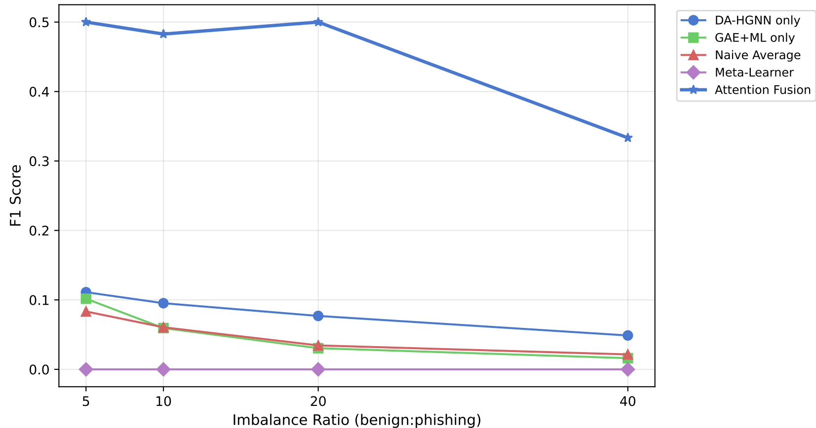
F1 Score vs Class Imbalance Ratio
