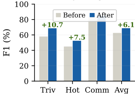
LLaDA-8B
