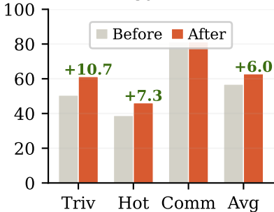
Dream-7B
