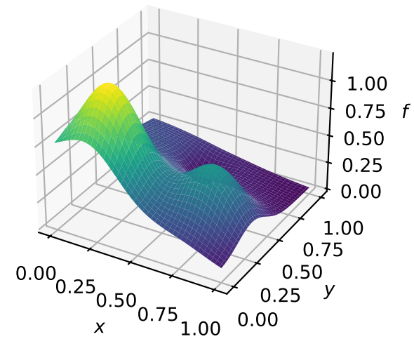
Franke function
