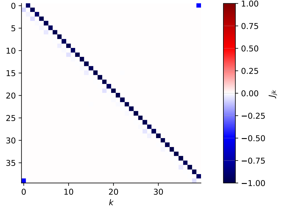
Lasso, \lambda = 0.01
