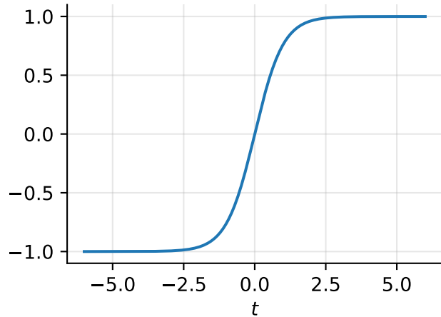
tanh
