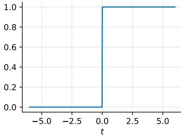
step
