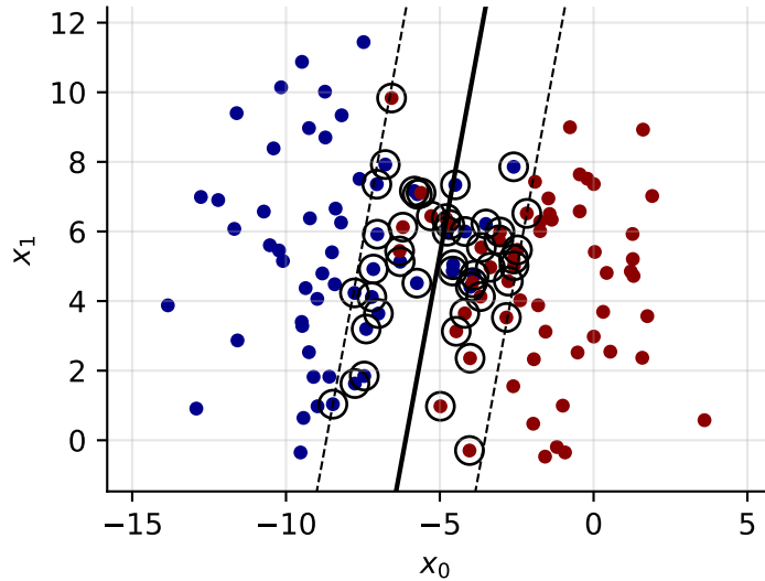
C = 0.01 : 48 SV, margin 5.05
