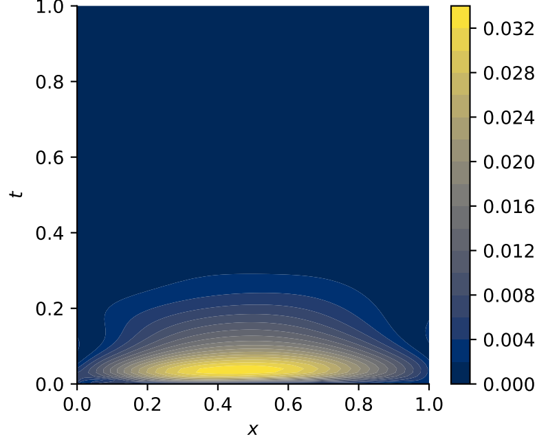
(b) PINN absolute error
