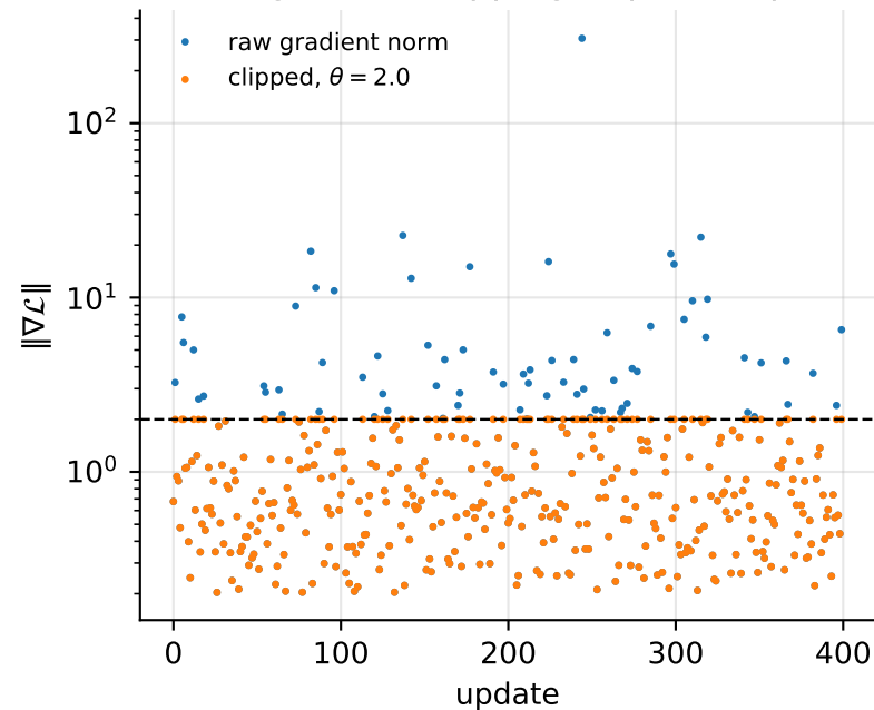
(c) gradient clipping, Eq. (11.clip)
