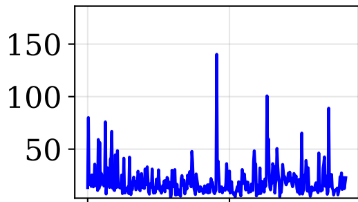
R-CNP
