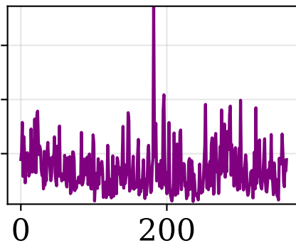
BLSTM
