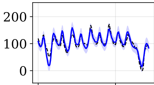
R-CNP
