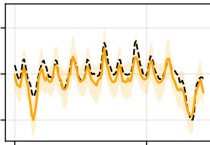
BLSTM
