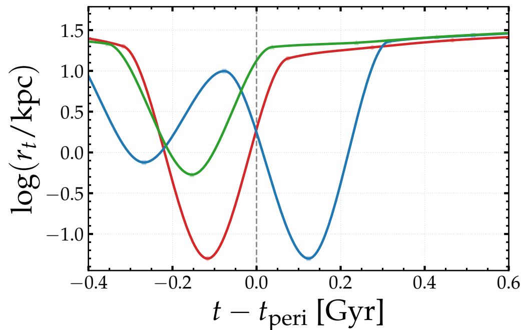
Tidal radius
