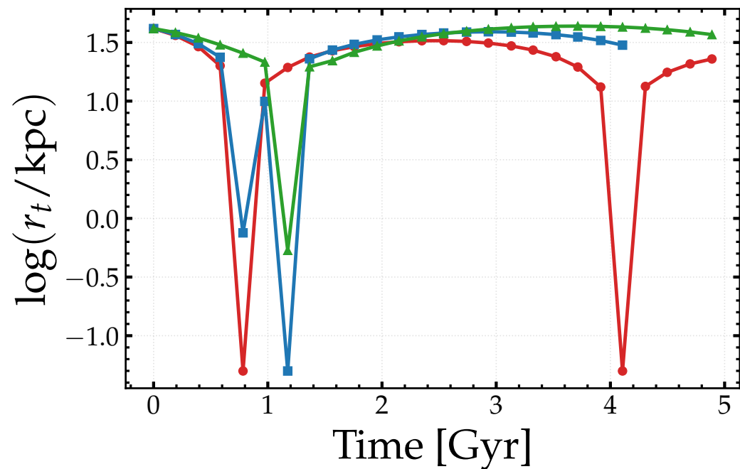
Tidal radius
