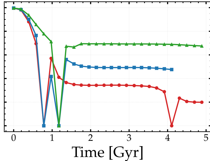
DM
