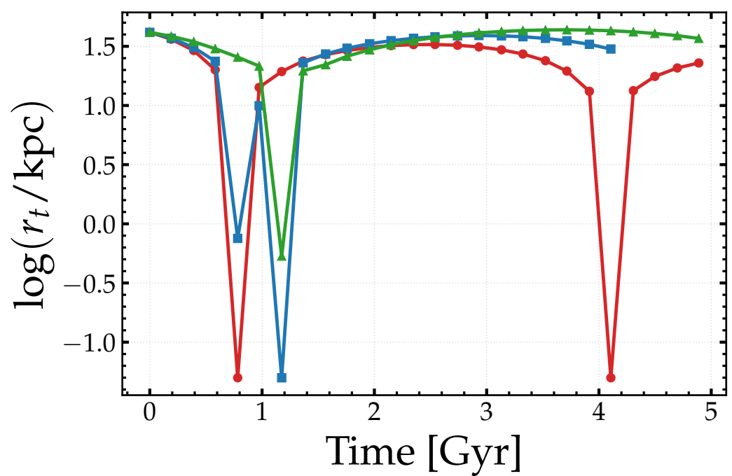
Tidal radius
