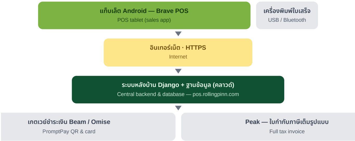
ภาพแสดงตัวอย่างการเชื่อมต่อของอุปกรณ์
