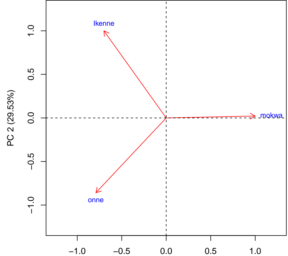
Biplot. Trait: TYLD
