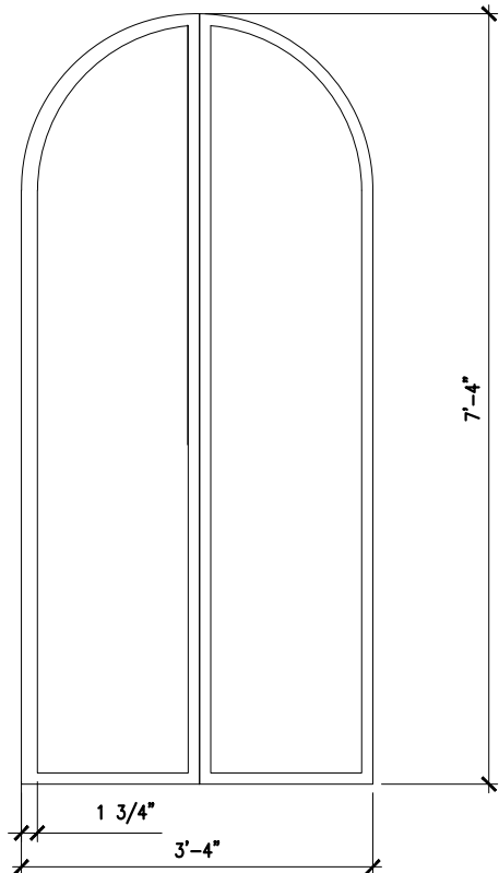
GLASS DOOR
