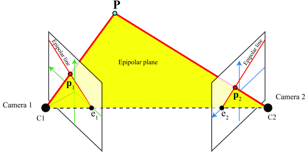
Figura 3: Modelo de la geometría epipolar para un solo punto.
