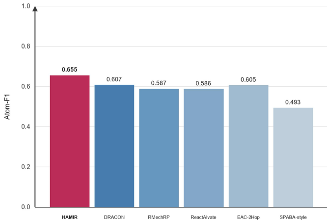
USPTO-MIT
