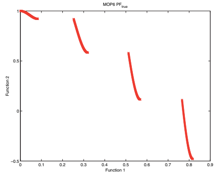
Fig. 4.12. MOP6 PF_{true}
