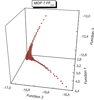
Fig. 4.14. MOP7 PF_{true}
