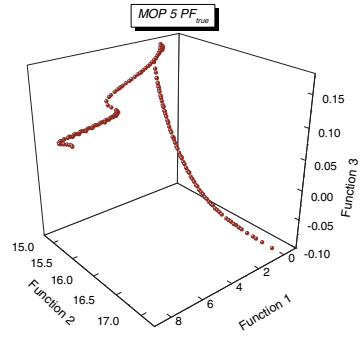
Fig. 4.10. MOP5 PF_{true}
