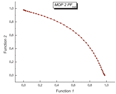
Fig. 4.4. MOP2 PF_{true}
