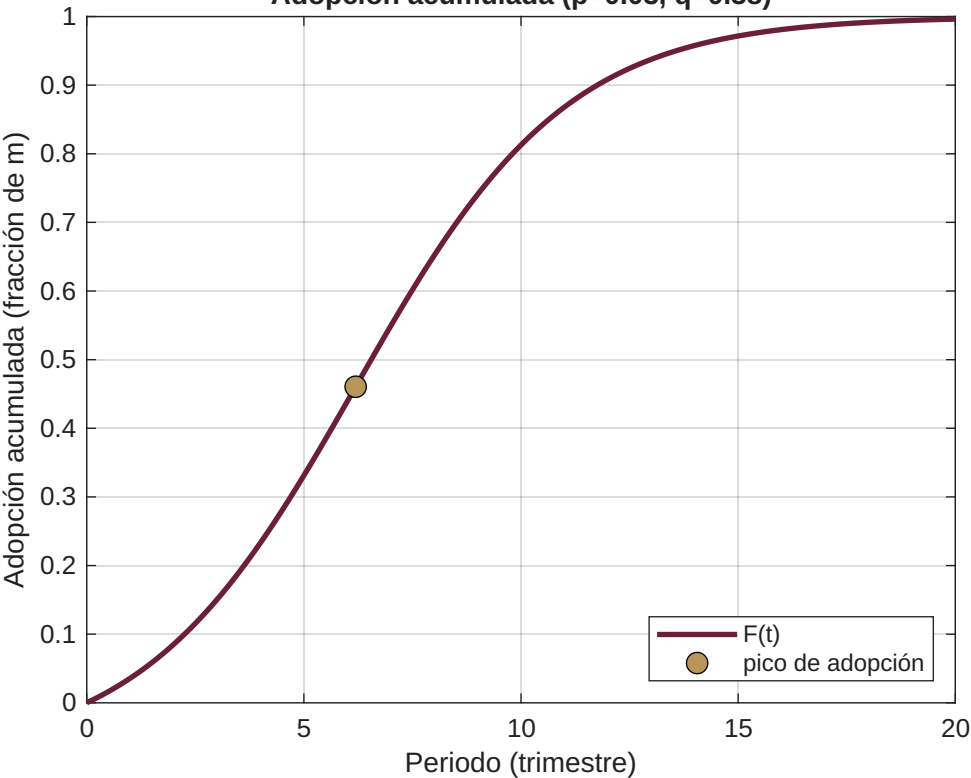
Adopción acumulada ( p=0.03 , q=0.38 )
