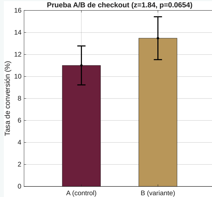
Figura 3.4: Prueba A/B de checkout: la versión B convierte 2.5 puntos porcentuales más, pero la diferencia no alcanza significancia estadística al 95 % ( p = 0,065 ). Fuente: elaboración propia con datos sintéticos.
