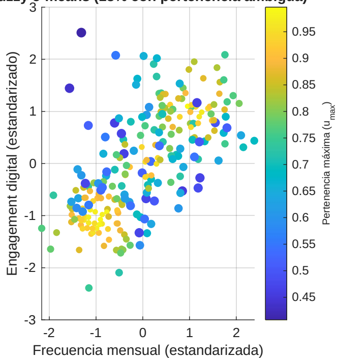
Fuzzy c-means (13% con pertenencia ambigua)
