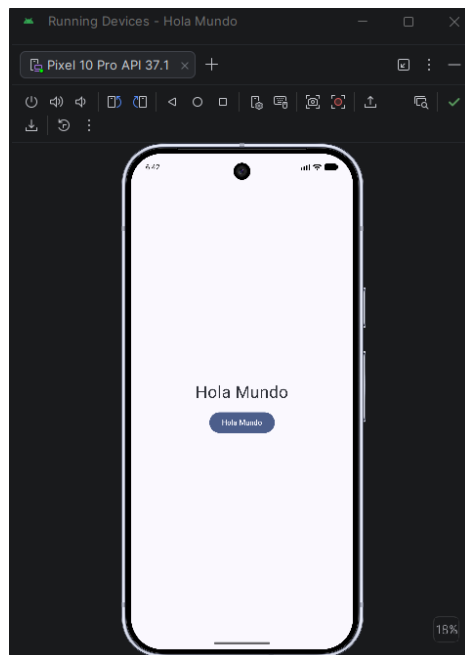
Ilustración 5. Programa ejecutado.
