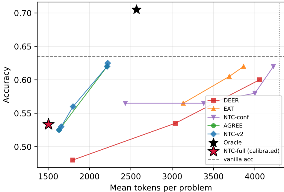
Qwen3-1.7B · math500 (n=200)
